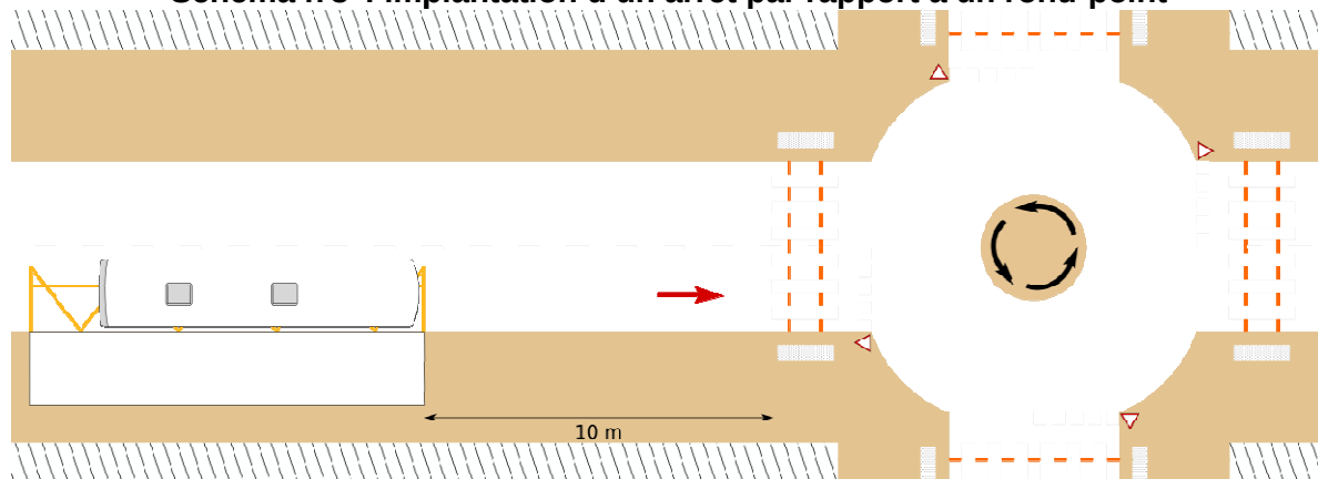
Schéma n°3 : implantation d'un arrêt par rapport à un rond-point
